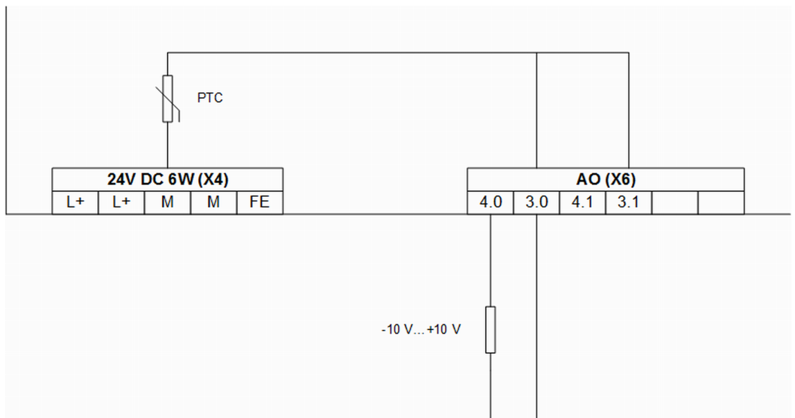
Fig. 80: Voltage output
