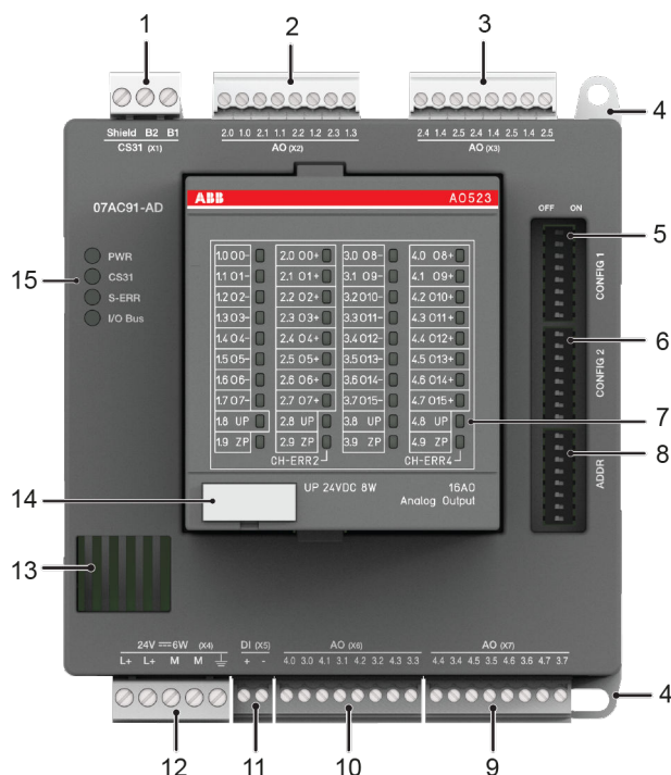
Fig. 67: Front view: 07AC91-AD
