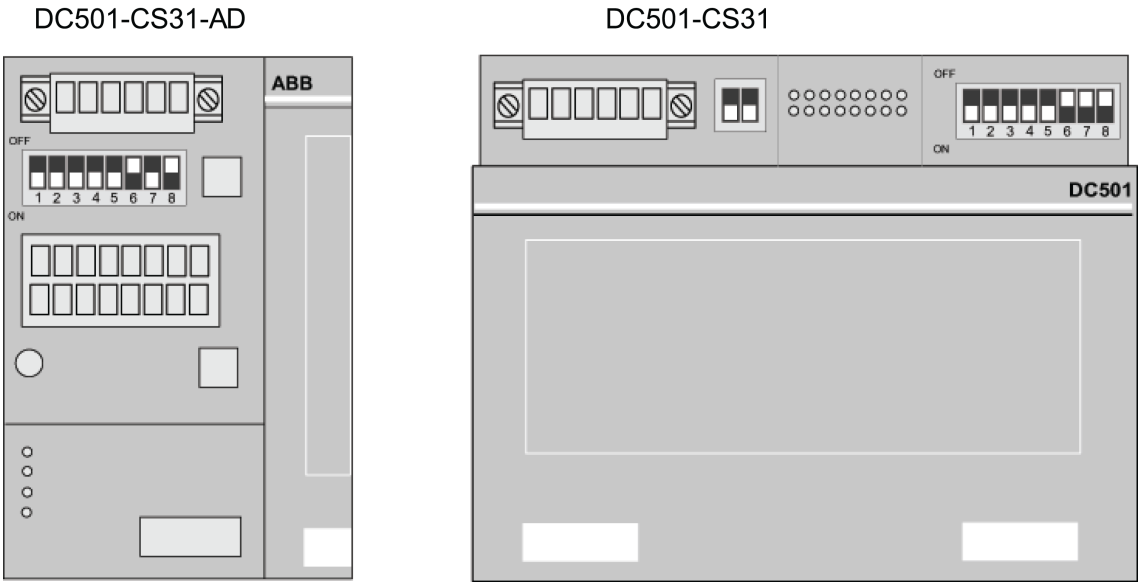
Fig. 95: DIP switch for DC501-CS31-AD
