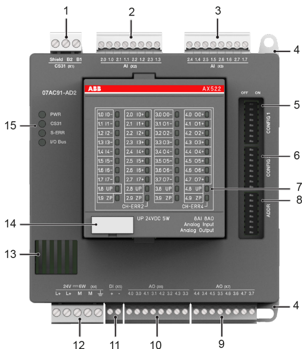
Fig. 75: Front view: 07AC91-AD2
