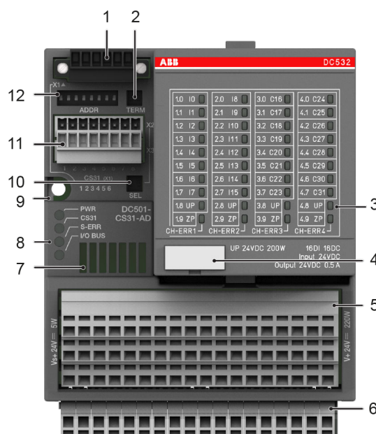
Fig. 85: Front view: DC501-CS31-AD
