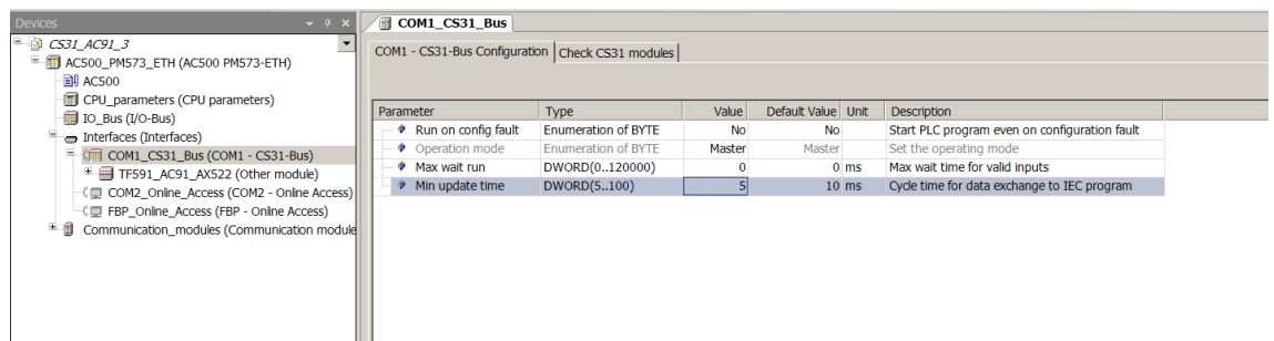
Fig. 12: Parameter configuration
