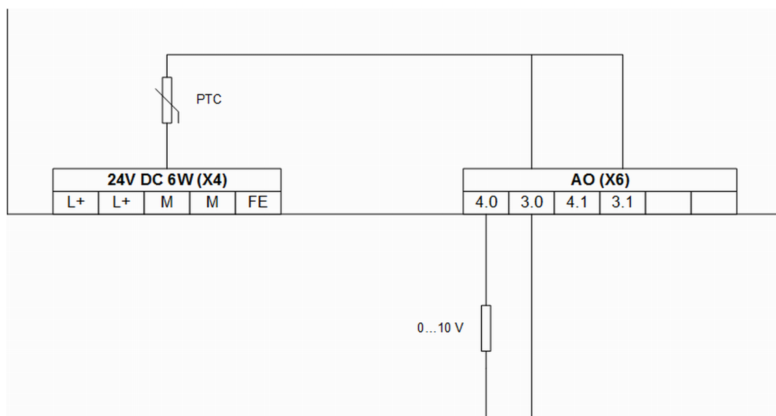
Fig. 70: Voltage output
