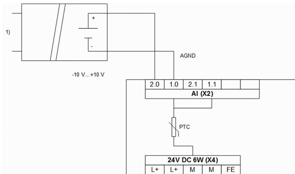
Fig. 78: Voltage input
