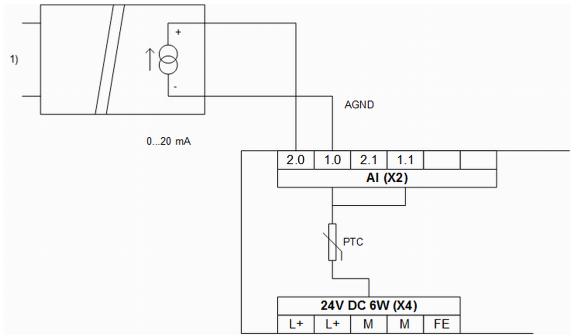
Fig. 79: Current input
