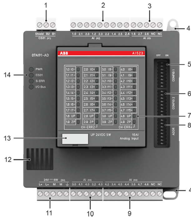
Fig. 56: Front view: 07AI91-AD
