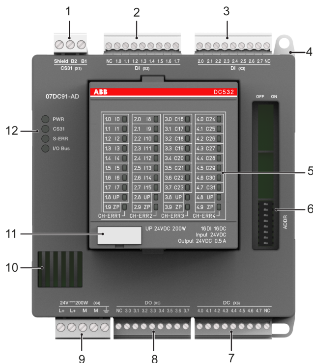
Fig. 37: 3ADR333196F0015_07DC91-AD_Front
