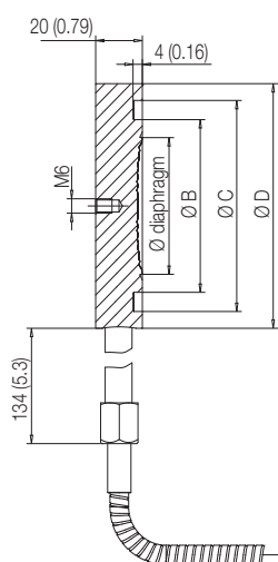
EN 1092-1 Form D
