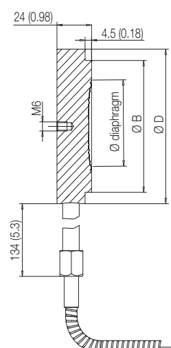
EN 1092-1 Form E
